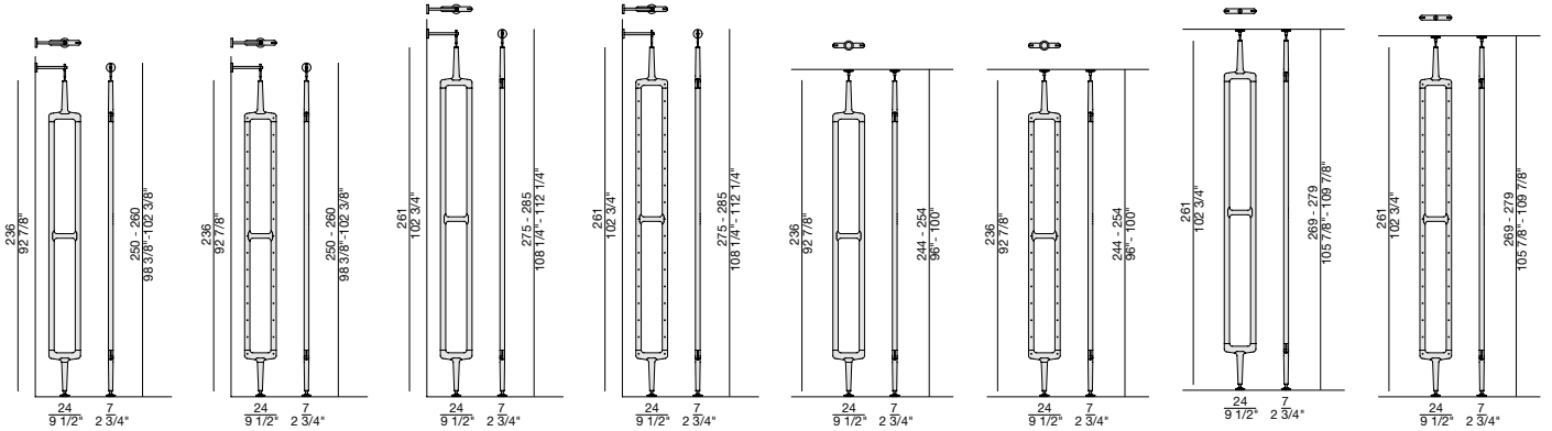
ARIA 236 COLONNA LATERALE A PARETE WALL SIDE COLUMN ARIA 236 COLONNA CENTRALE A PARETE WALL CENTRAL COLUMN ARIA 261 COLONNA LATERALE A PARETE WALL SIDE COLUMN ARIA 261 COLONNA CENTRALE A PARETE WALL CENTRAL COLUMN ARIA 236 COLONNA LATERALE A SOFFITTO CEILING SIDE COLUMN ARIA 236 COLONNA CENTRALE A SOFFITTO CEILING CENT. COLUMN ARIA 261 COLONNA LATERALE A SOFFITTO CEILING SIDE COLUMN ARIA 261 COLONNA CENTRALE A SOFFITTO CEILING CENT. COLUMN
