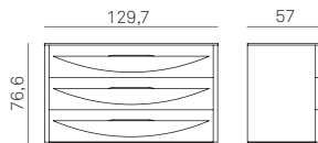
Elemento 3 cassetti P=57 H=76,6
