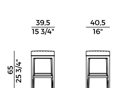
695/S sgabello basso \ counterstool
