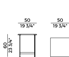
878/TQ-50 tavolino \ coffee table
