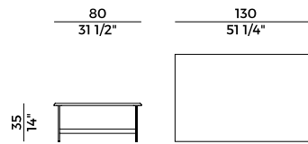
878/TR tavolino \ coffee table
