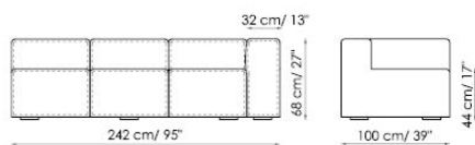
Divano angolare 242 Corner sofa Prof. 100 depth dx right
