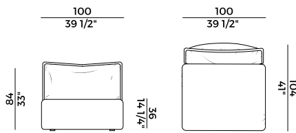
935/DM1 modulo centrale \ central unit
