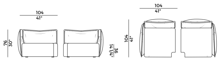
935/DA-90° modulo angolare destro e sinistro \ right and left corner unit
