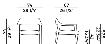
906/PLI poltrona \ lounge chair
