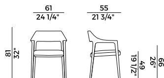
906/P poltroncina \ armchair
